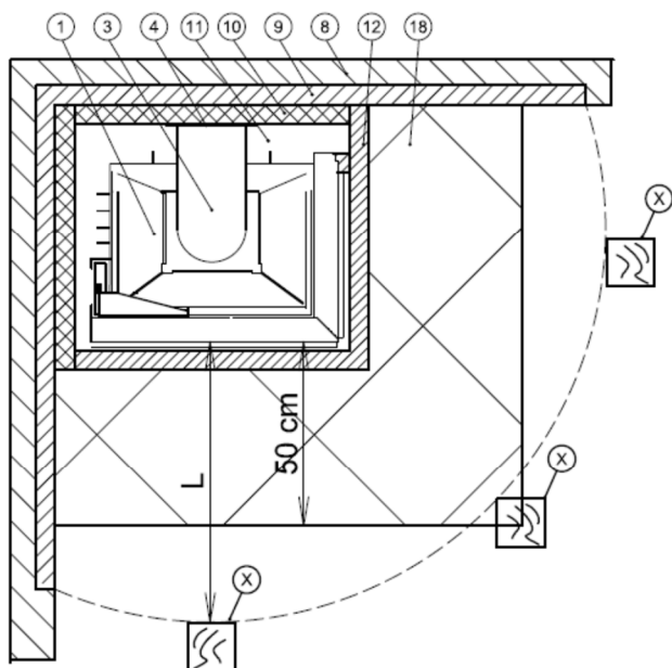
Abb. 3.2. Beispiel eines Einsatzes mit zweiseitiger Verglasung
