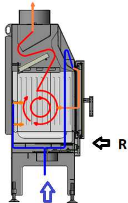
Abb. 4.3. Luftzirkulation:
