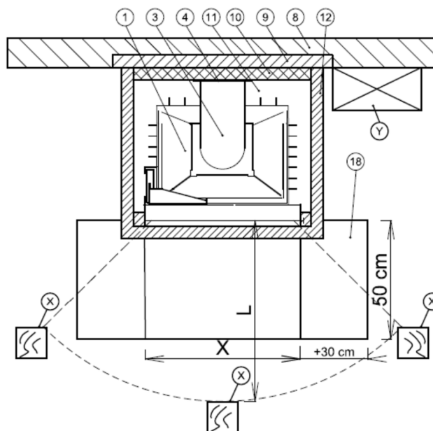
Abb. 3.3. Beispiel eines Einsatzes mit Frontverglasung
