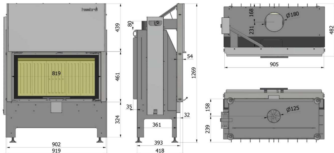
Abb. 2.17. Heatro 81H
