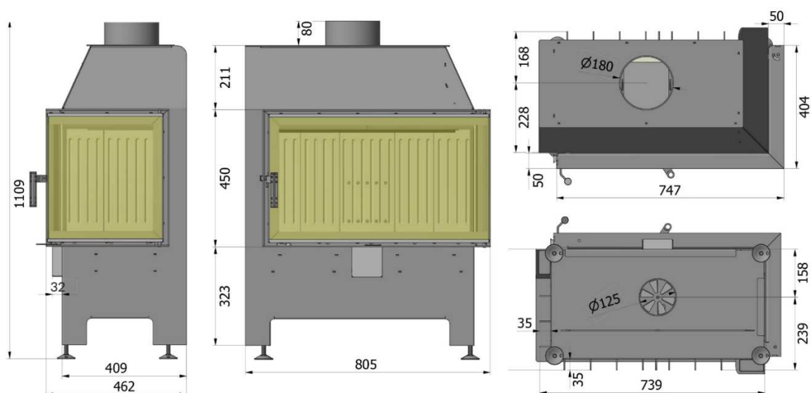
Abb. 2.10. Heatro 69P
