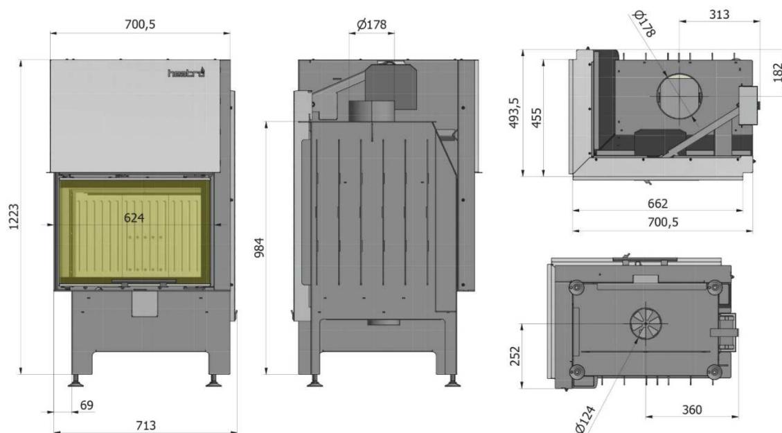
Abb. 2.6. Heatro 55LH
