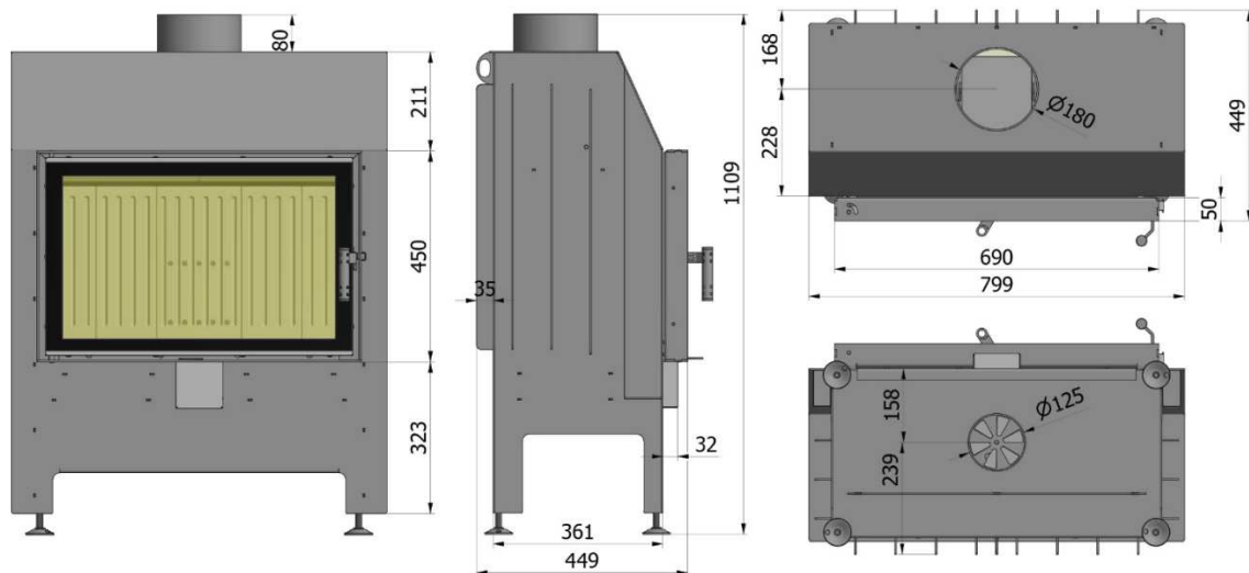
Abb. 2.8. Heatro 69
