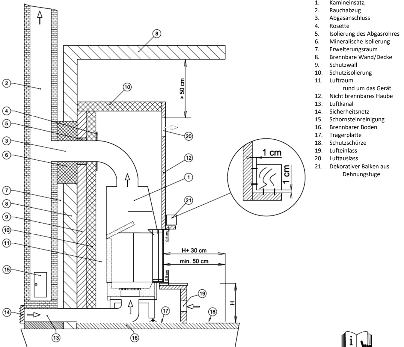
Abb. 3.1. Beispiel für die Geräteinstallation
