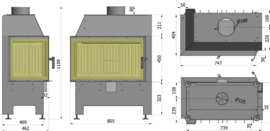
Abb. 2.9. Heatro 69L
