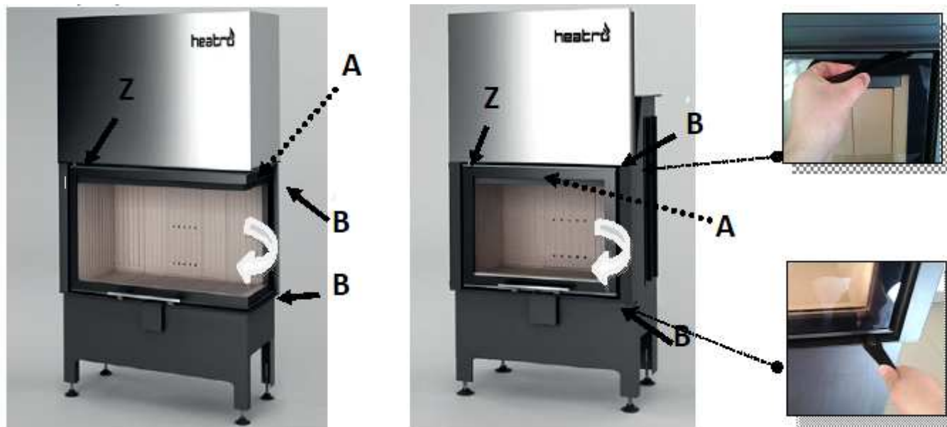
Abb. 4.1. So öffnen Sie die Tür zum Reinigen
