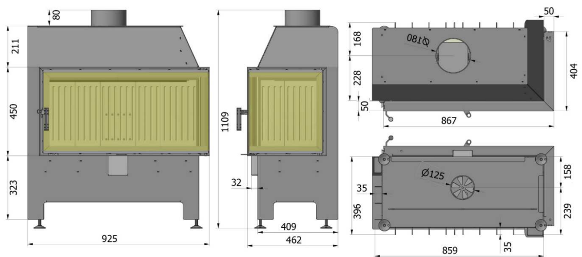
Abb. 2.16. Heatro 81P
