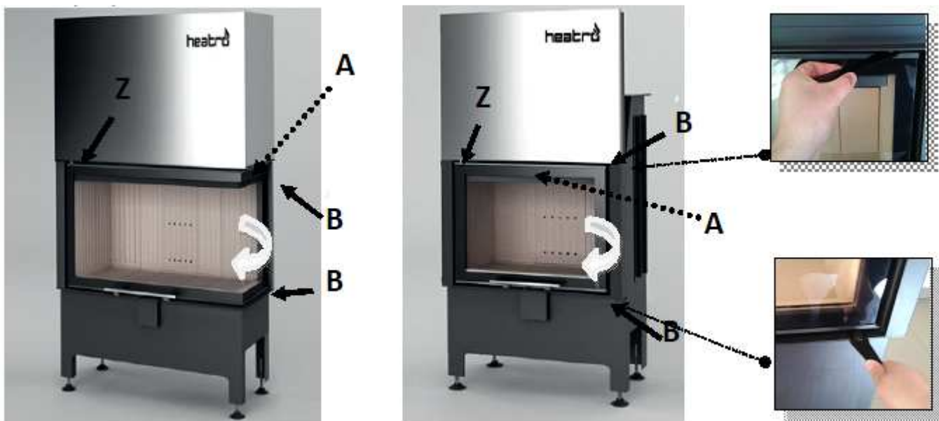
Abb. 4.4. Öffnen der Reinigungstür bei der Ausführung mit Türliftsystem
