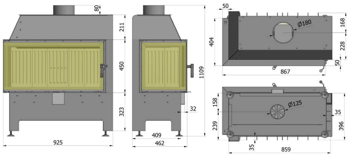
Abb. 2.15. Heatro 81L
