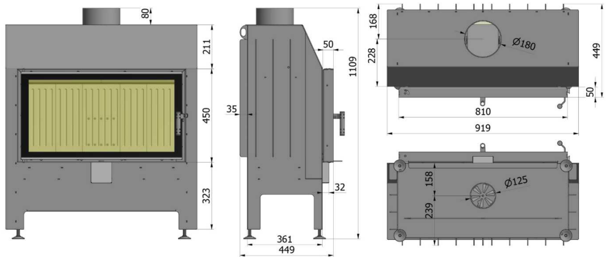
Abb. 2.14. Heatro 81
