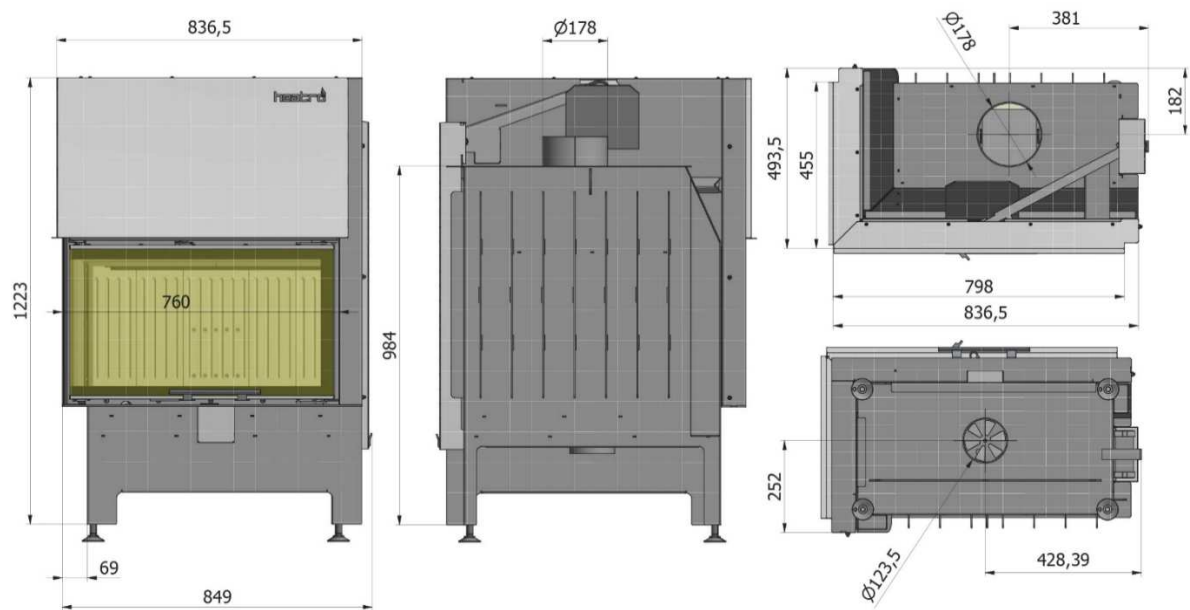
Abb. 2.12. Heatro 69PH
