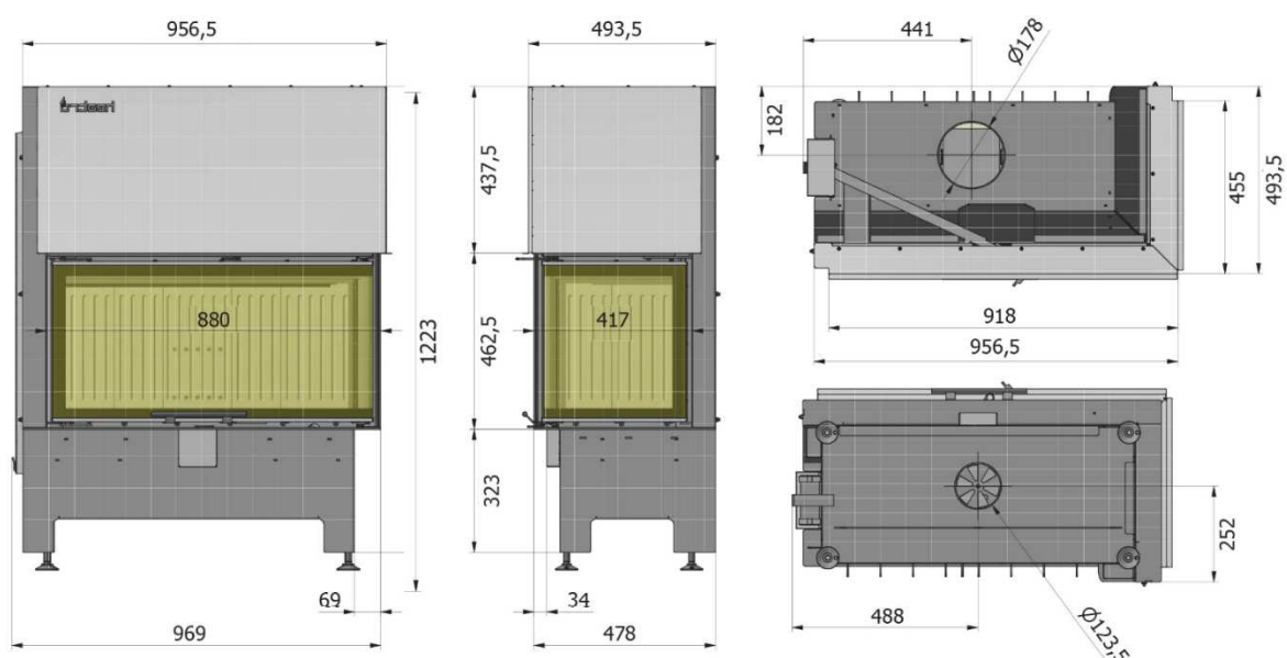
Abb. 2.19. Heatro 81PH
