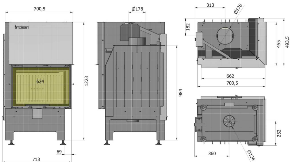
Abb. 2.7. Heatro 55PH
