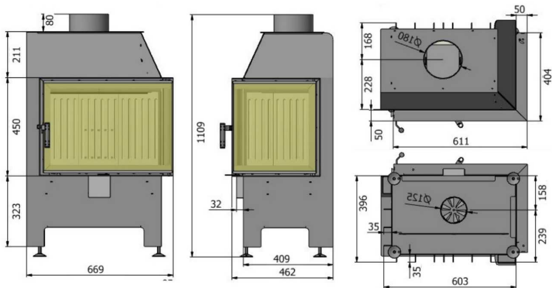
Abb. 2.4. Heatro 55P
